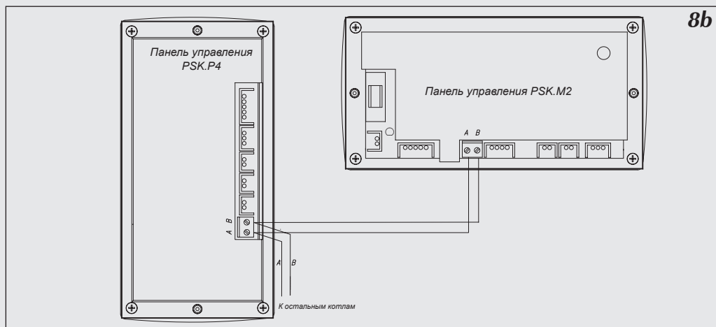
Рис.8b Подключение панелей управления группы котлов.
