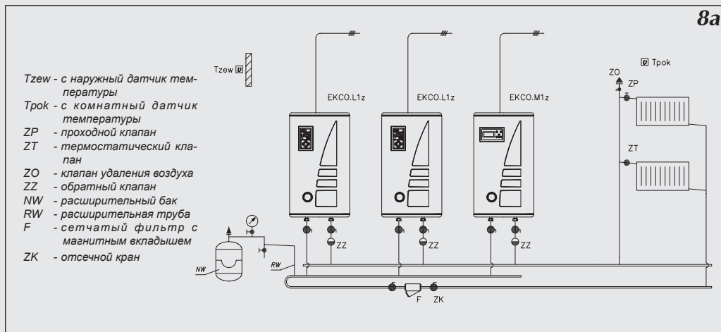
Рис.8а Подключение группы котлов.
