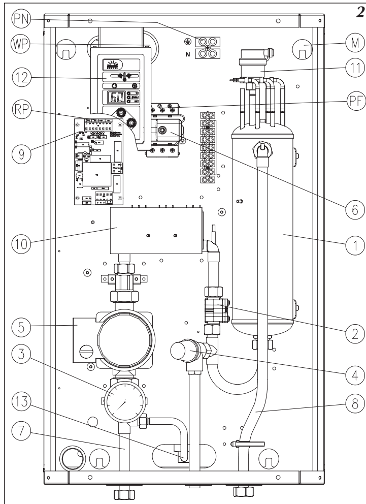
Рис.2 Конструкция котла ЕКСО.L1N
