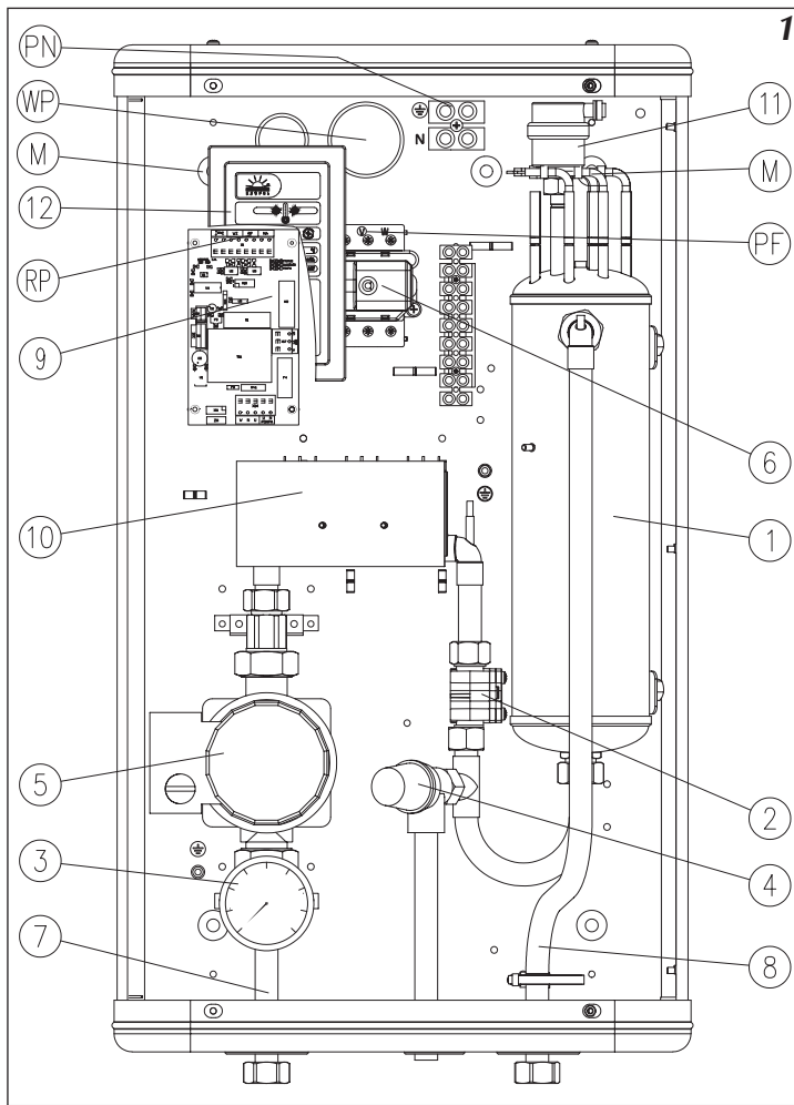
Рис.1 Конструкция котла ЕКСО.1.1
