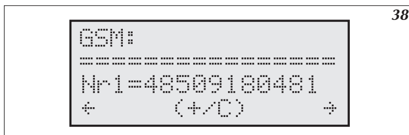
Рис.38 Дисплей установки телефонов, имеющих допуск к управлению котлом.
