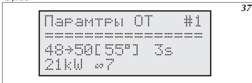
Рис.37 Страница общего просмотра при групповой работе котлов.
