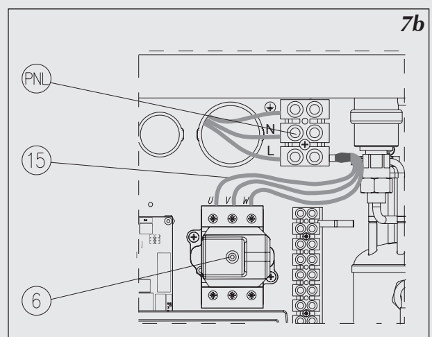
Рис.7b Подключение котла к однофазной сети (касается мощностей 4кВт, 6 кВт и 8 кВт)
