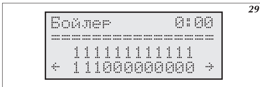
Рис.29 Страница теплообменник – суточная программа.
