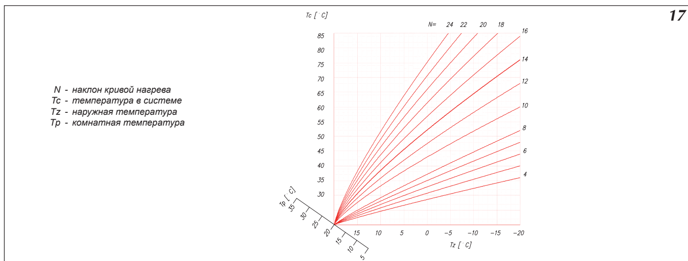
Рис. 17 Кривая нагрева
