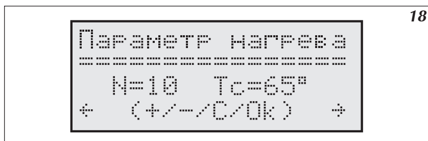
Рис. 18 Страница установки кривой нагрева
