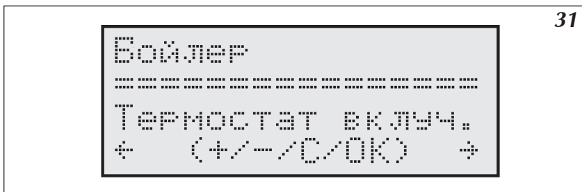
Рис.31 Страница „Теплообменник – измерение температуры при помощи термостата”
