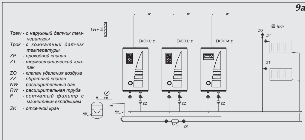
Рис.9а Подключение группы котлов.
