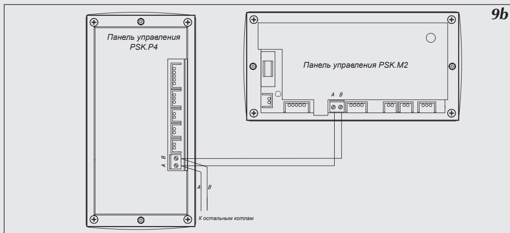
Рис.9b Подключение панелей управления группы котлов.
