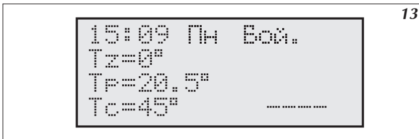
Рис.13 Общий обзор при конфигурации „ОТ.НЕТ ВОД.ДА” (выключен обогрев отопительной системы и включен контур обогрева теплообменника)
