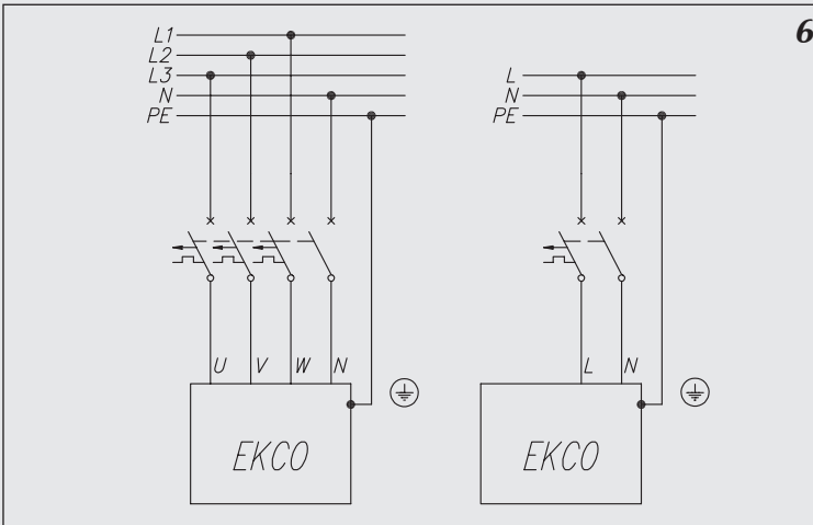
Рис.6 Подключение к электросети
