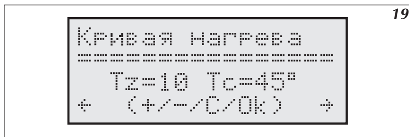
Рис.19 Страница актуальной кривой нагрева
