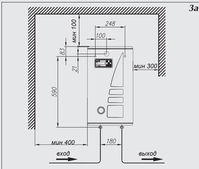
Рис.3а, 3б Эскиз крепления котла на стене.
