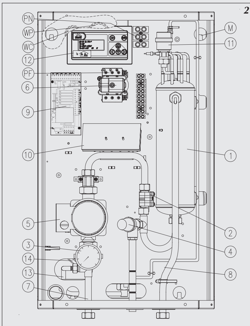
Рис.2 Конструкция трехфазного котла ЕКСО.М1Nz
