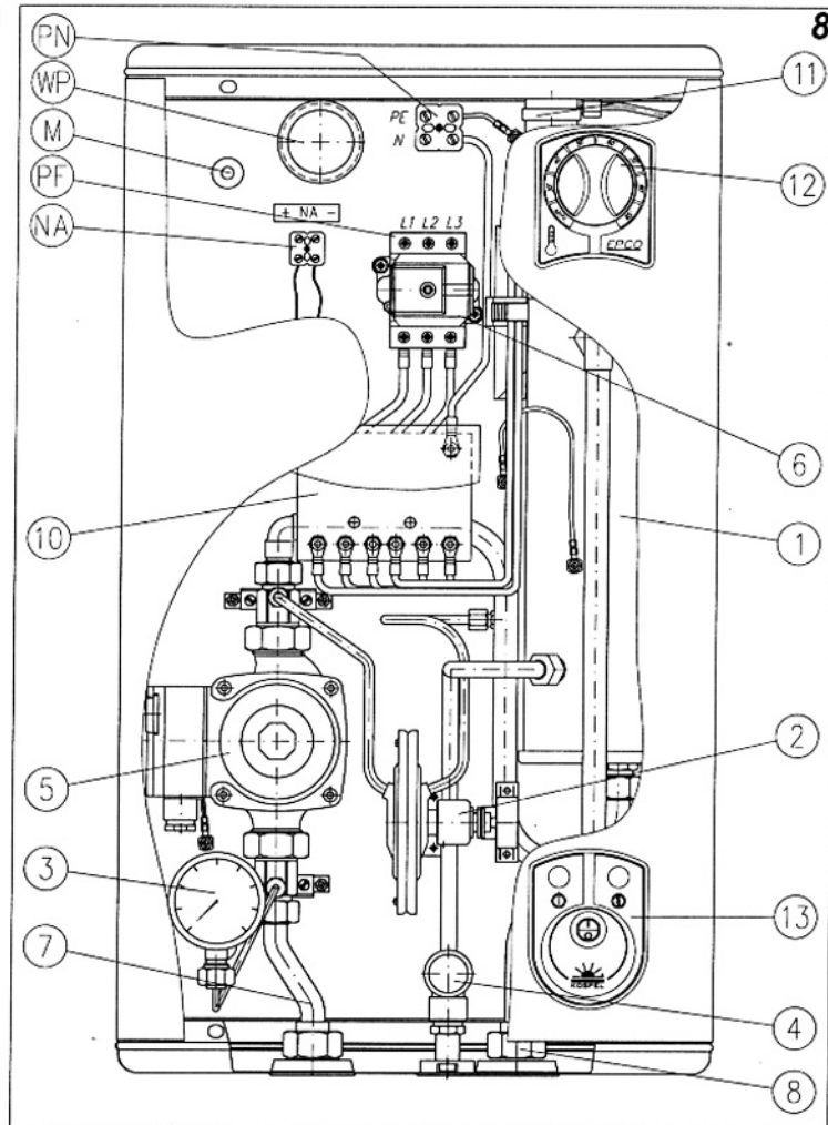
Рис.8 Устройство трёхфазного котла
